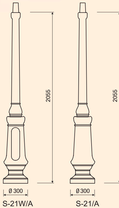
słup S-21W/A, układ ramion 2 w górę, oprawy OP E/Z/400, klosze Kule mrożone Ø 400
