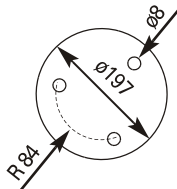
podstawka z rozstawem otworów mocujących
