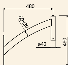
Kinkiet KA-C1, oprawa OPA, klosz Kula przezroczysta Ø400, raster ze stali nierdzewnej
